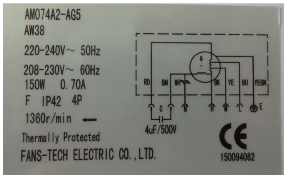
Fan motor
