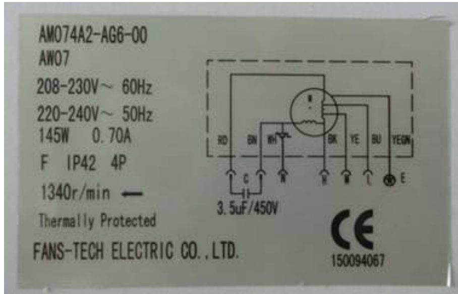
Fan motor
