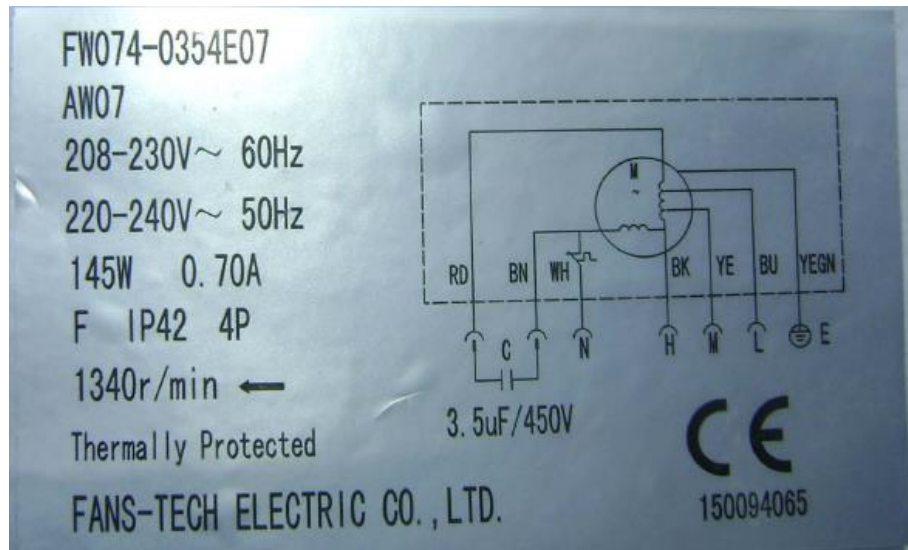
Fan motor
